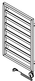
Billo EBL 530x830 konfiguracja prawa rys. aksjometryczny
